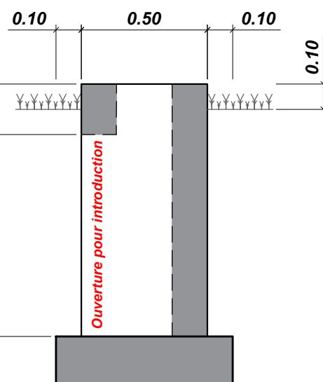
Coupe B-B'
